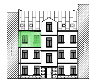
Elewacja tylnia
